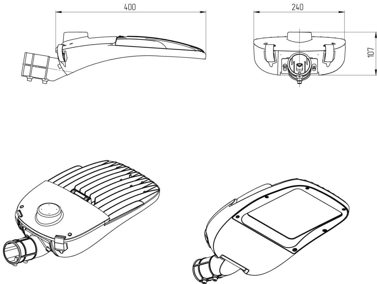
Рисунок 1. Общий вид светильника RAD-TURBO
