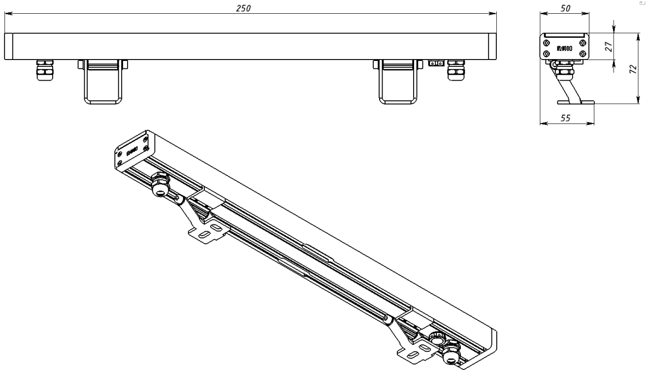
Рисунок 1. Общий вид светильника RAD-L-ST
