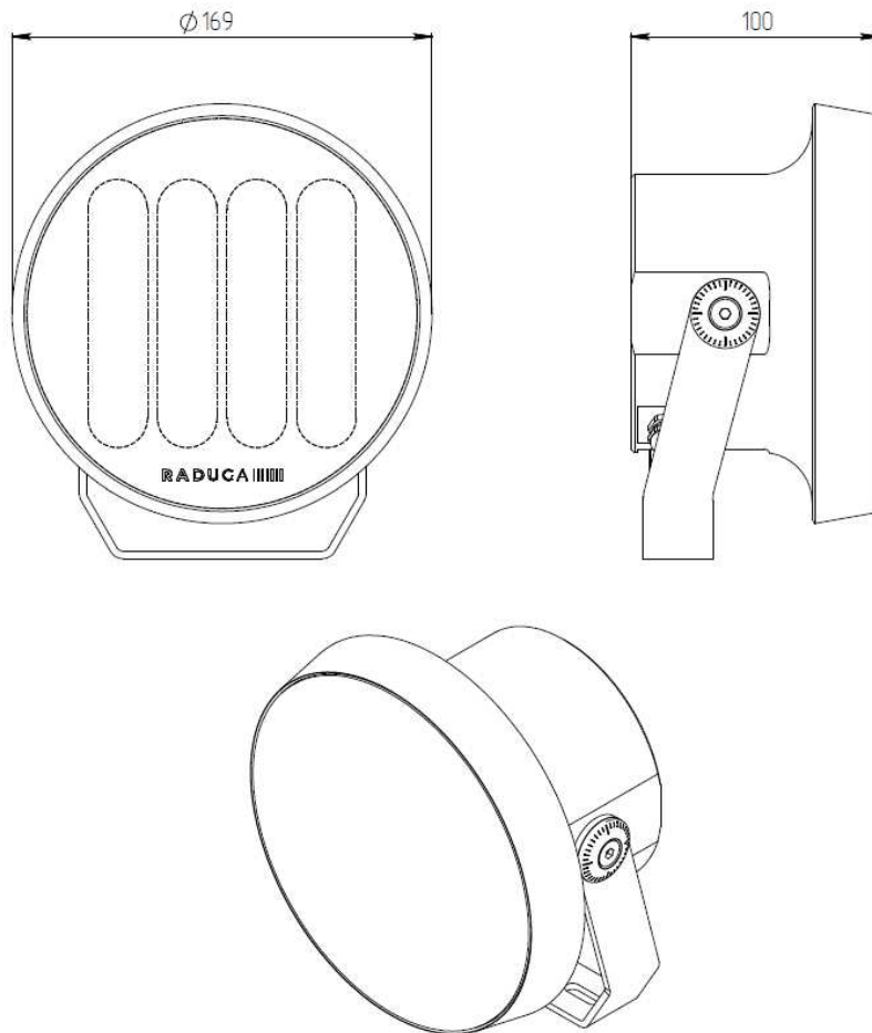
Рисунок 1. Общий вид светильника RAD-S-CLM
